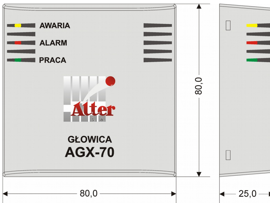
Rys.1. Widok i podstawowe wymiary głowic AGX-70
