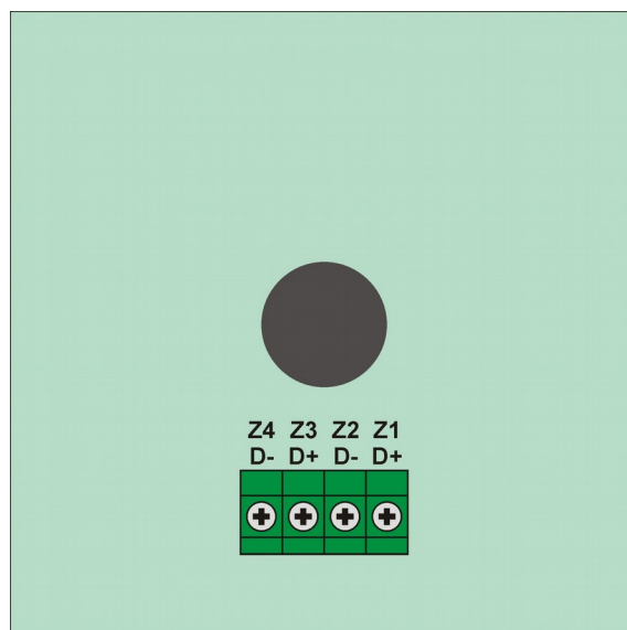
Rys.3. Widok zacisków przyłączeniowych głowic AGX-70
