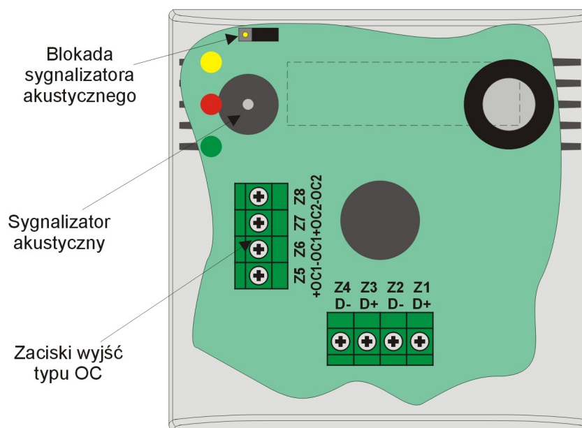
Rys.4. Rozmieszczenie opcjonalnych elementów w obudowie głowicy
