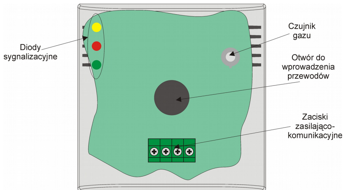
Rys.2. Podstawowe elementy głowic AGX-70
