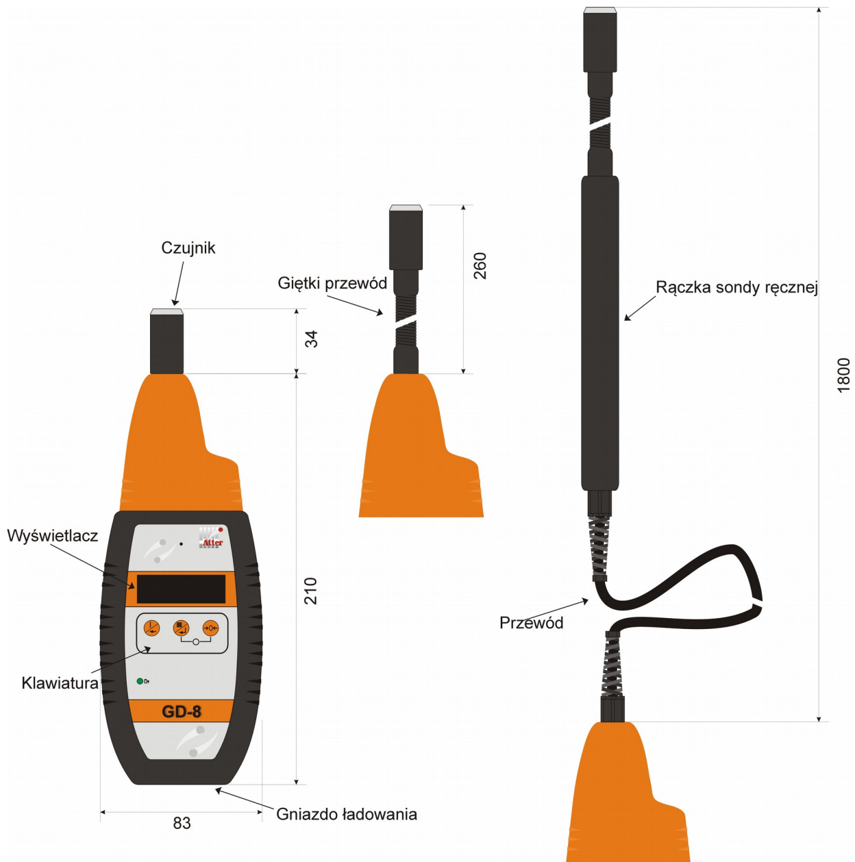
Rys.1. Widok i podstawowe wymiary w zależności od posiadanej wersji (wymiały podane w mm)
