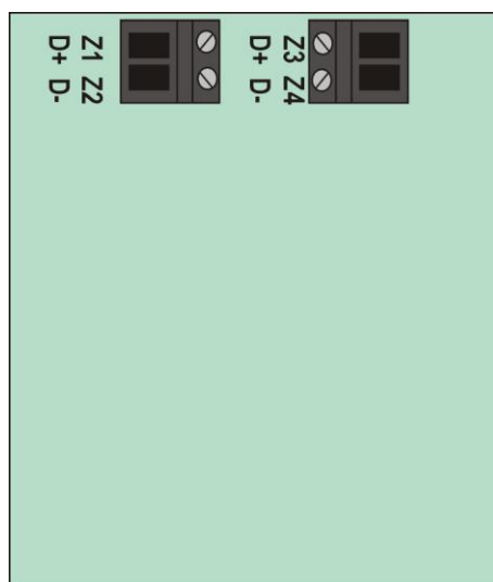
Rys.6. Widok zacisków przyłączeniowych głowic GDY-70
