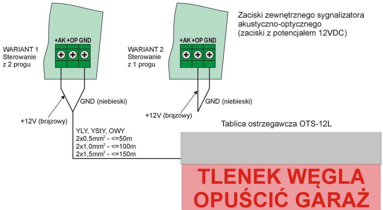
Rys.3. Przykłady podłączania tablicy OTS-12L do wyjść sygnalizatora akustyczno-optycznego
