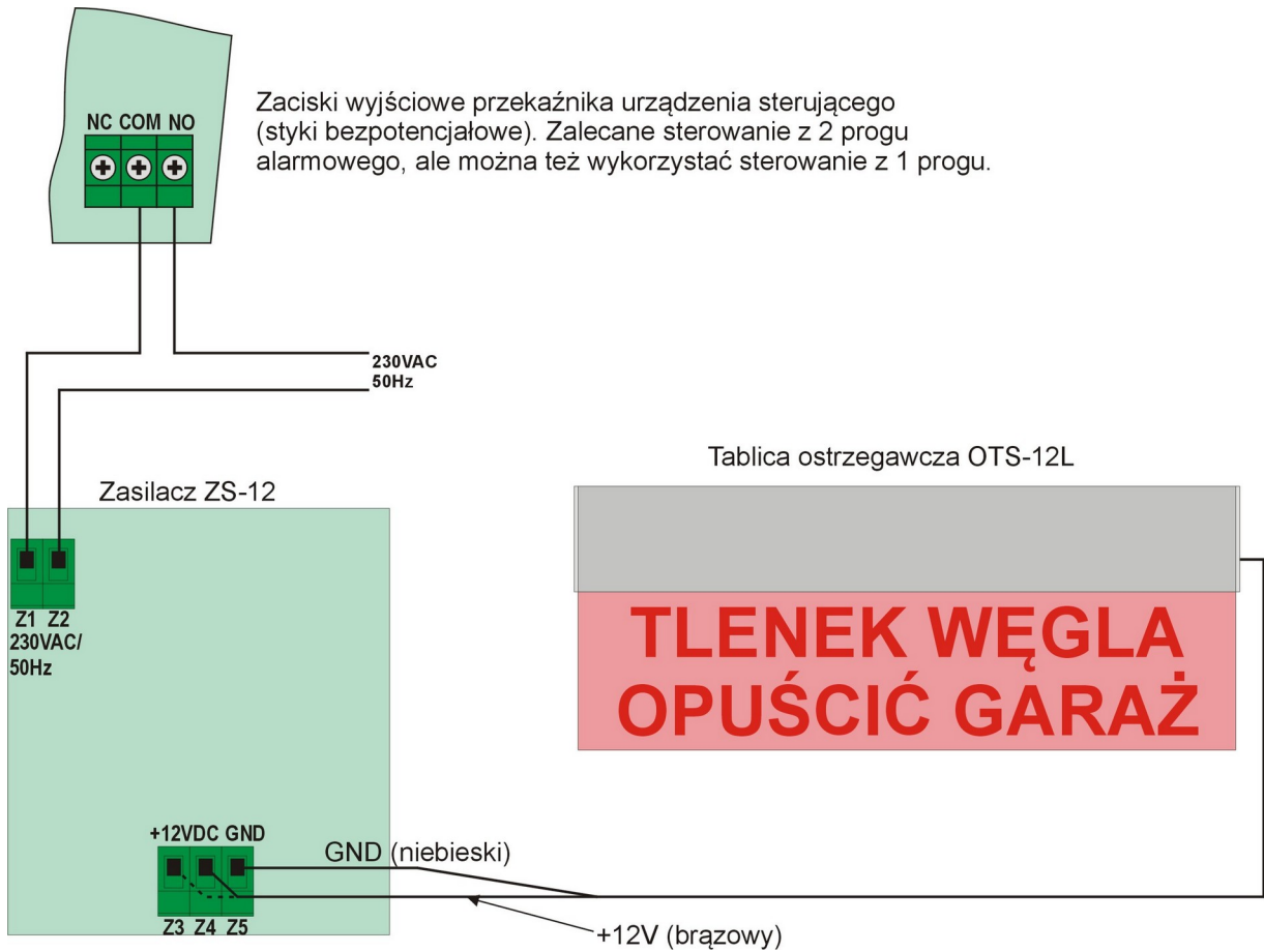
Rys.2. Przykład podłączania tablicy OTS-12L do bezpotencjałowych wyjść przekaźnikowych
