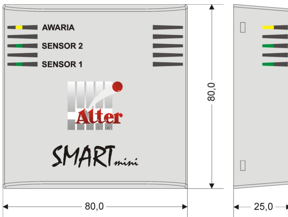
Rys.51. Widok i podstawowe wymiary głowic SMARTmini
