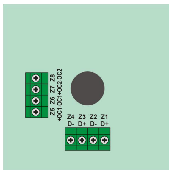
Rys.52. Widok zacisków przyłączeniowych głowic SMARTmini
