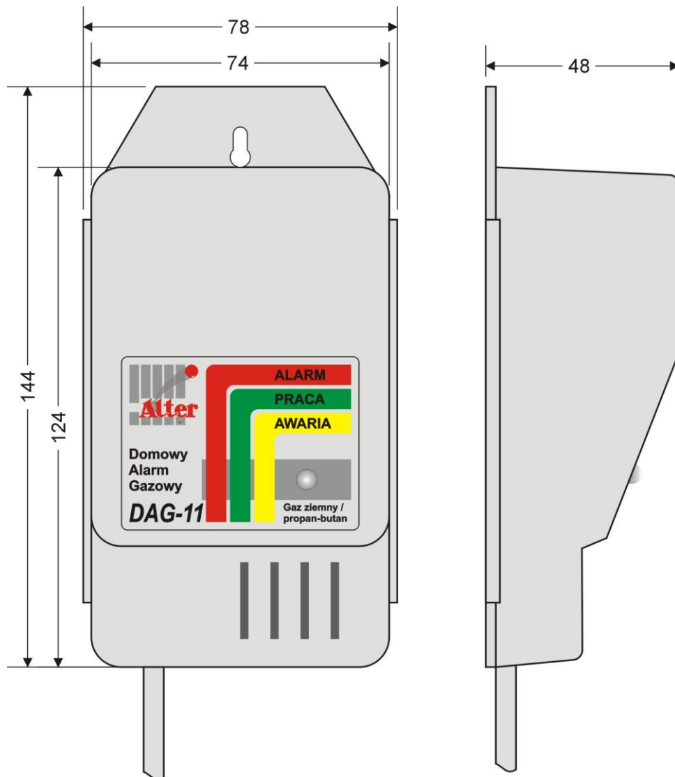
Rys.1. Widok i podstawowe wymiary DAG-11
