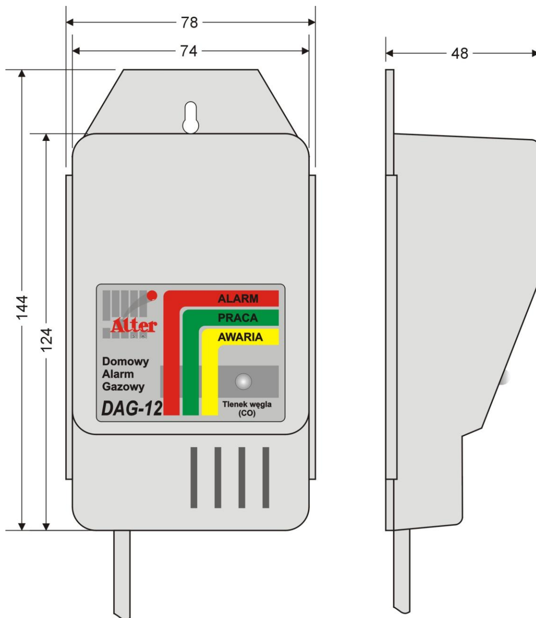
Rys.1. Widok i podstawowe wymiary DAG-12
