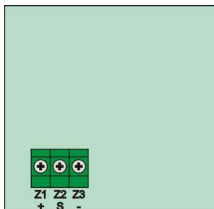
Rys.31. Widok zacisków głowicy GD-73
