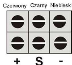
Rys.30. Widok zacisków głowic GD-71 i GD-72
