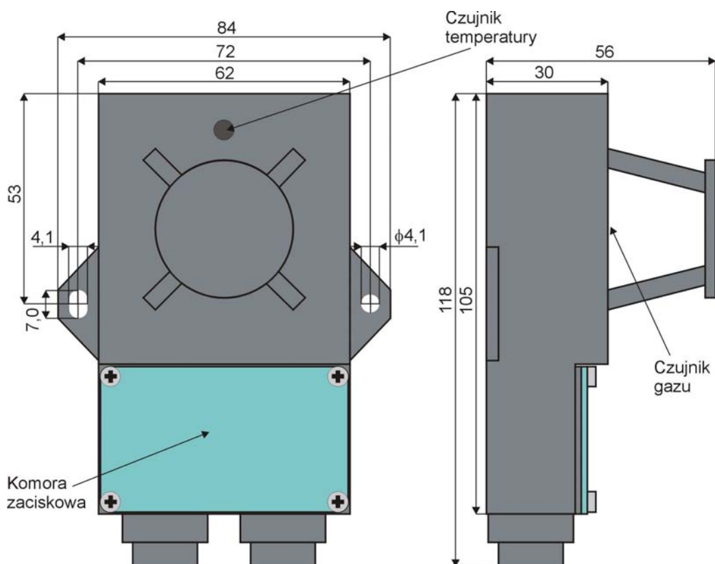
Rys.28. Widok i podstawowe wymiary głowic detekcyjnych GD-71 i GD-72
