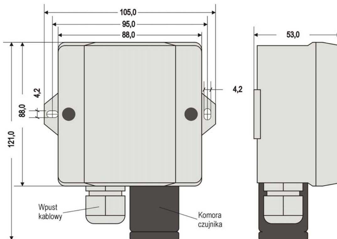
Rys.29. Widok i podstawowe wymiary głowic detekcyjnych GD-73
