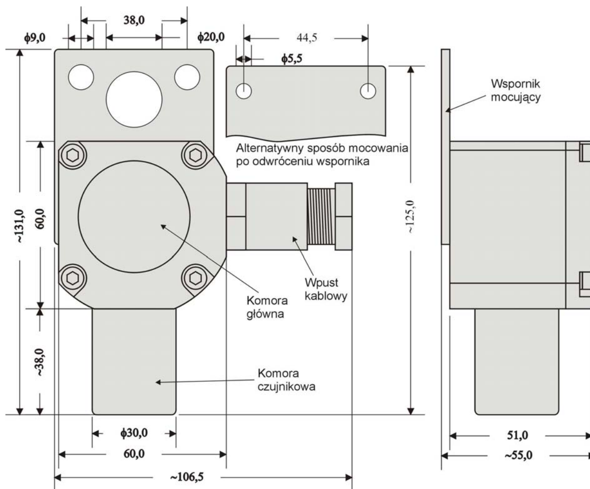
Rys.32. Widok i podstawowe wymiary głowic detekcyjnych GD-21
