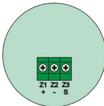
Rys.33. Widok zacisków głowicy GD-21
